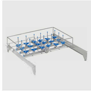
C713 : 上段バスケット18ジェット mm.80/110h ø mm.6
