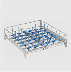
C711 : 上段バスケット36ジェット mm.80/110h ø mm.6
